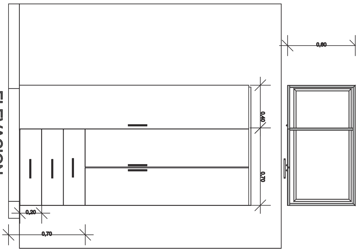
PLANTA
