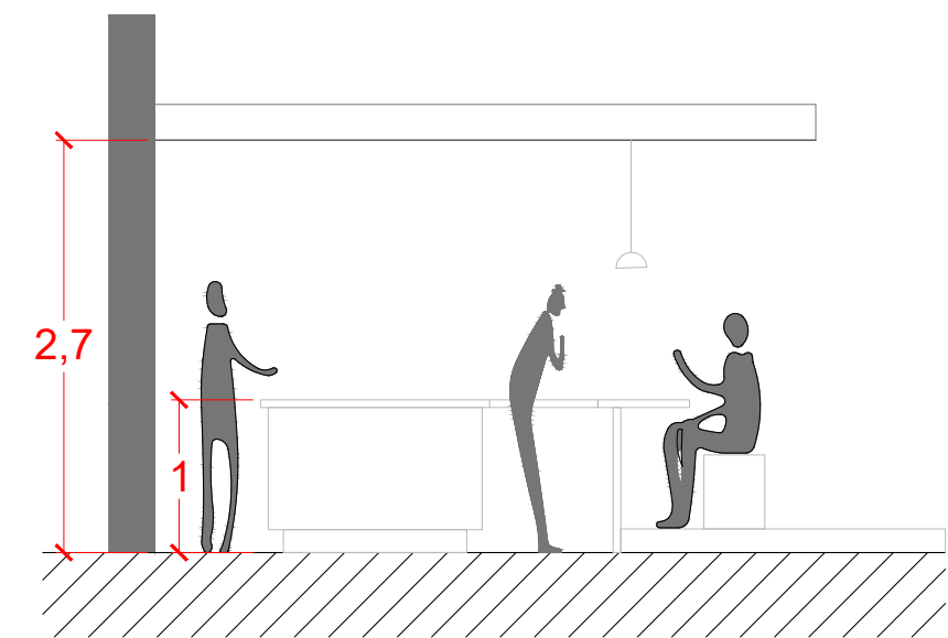
Sección Transversal
